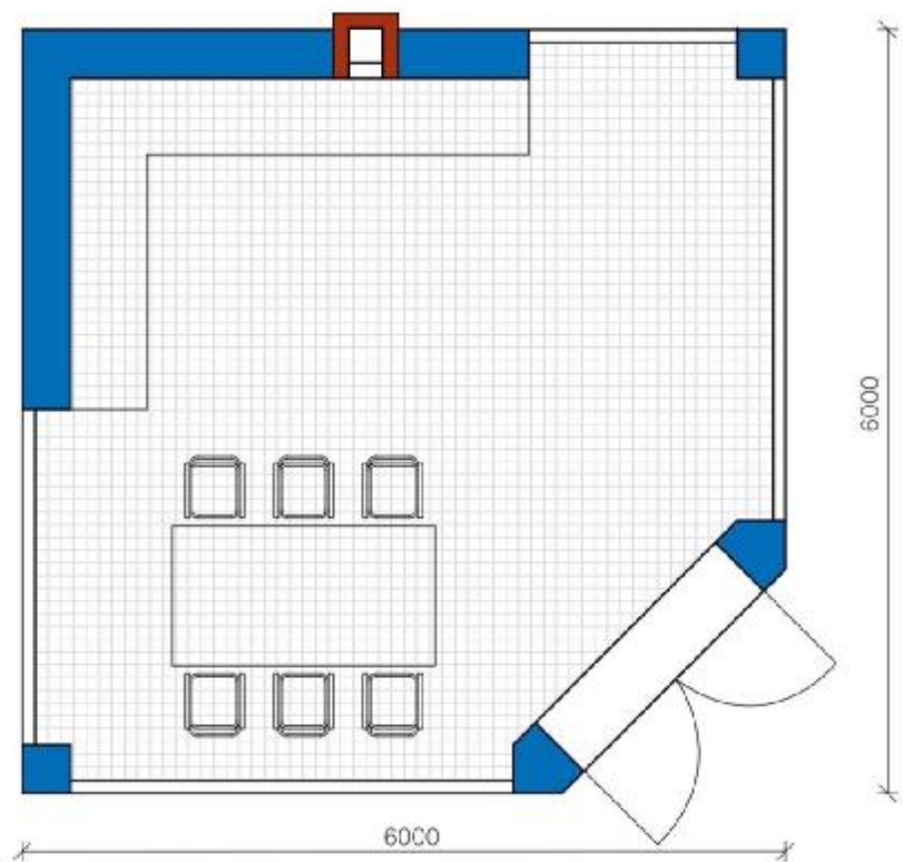
План беседки
