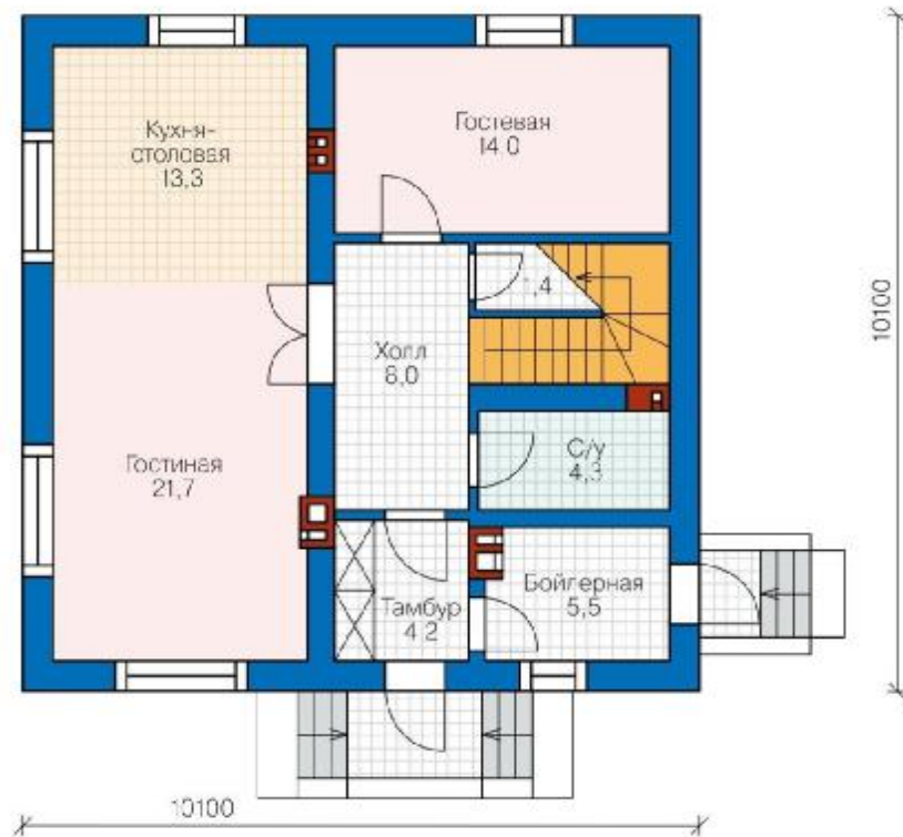
План первого этажа
