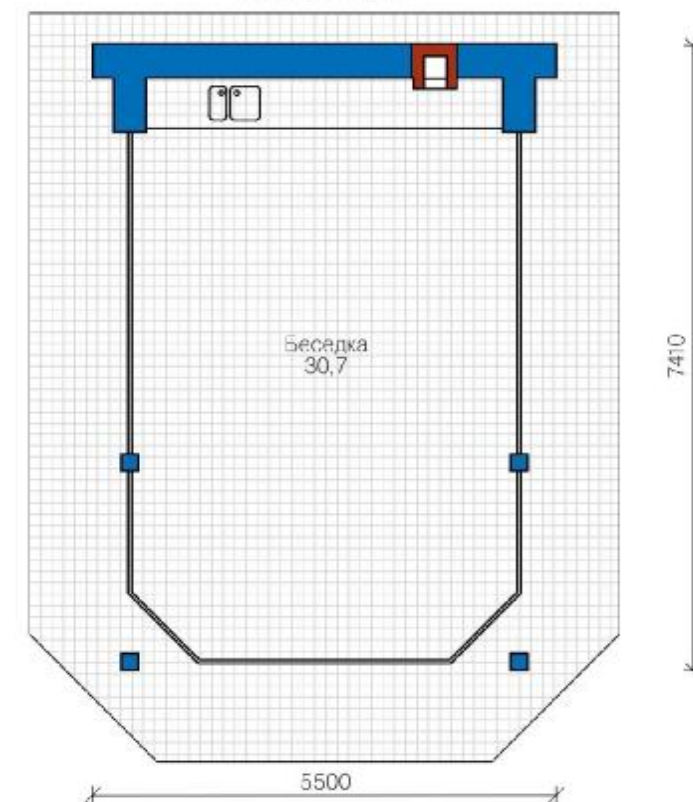
План беседки
