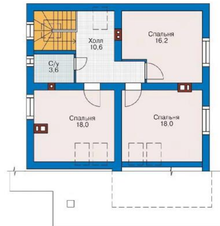
План мансардного этажа
