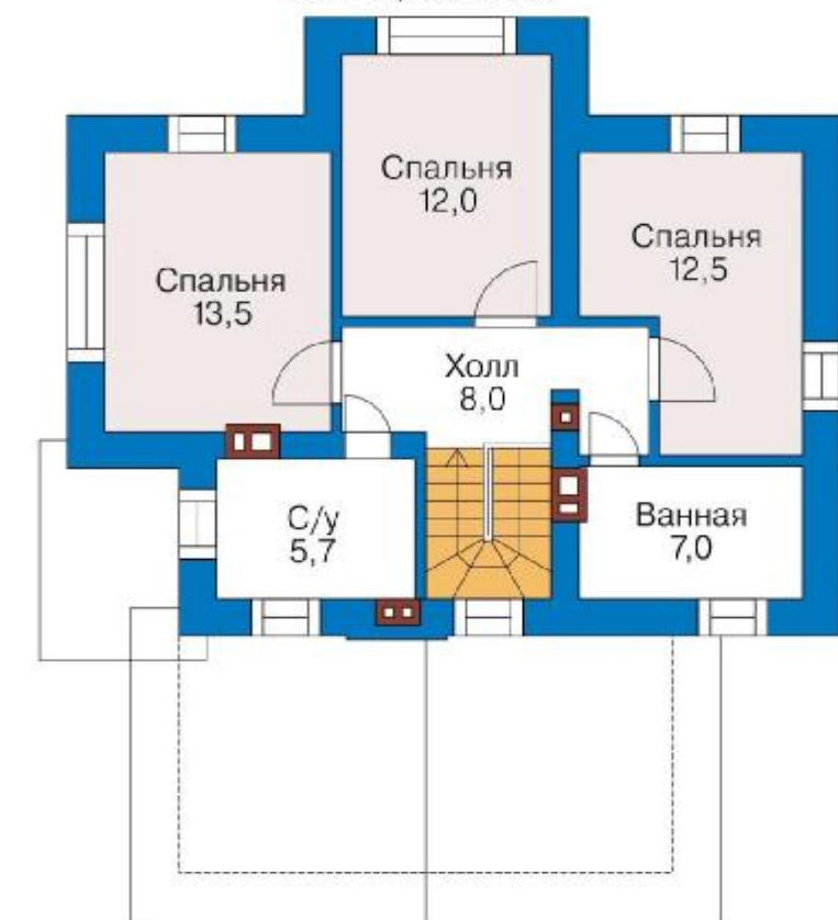
План второго этажа
