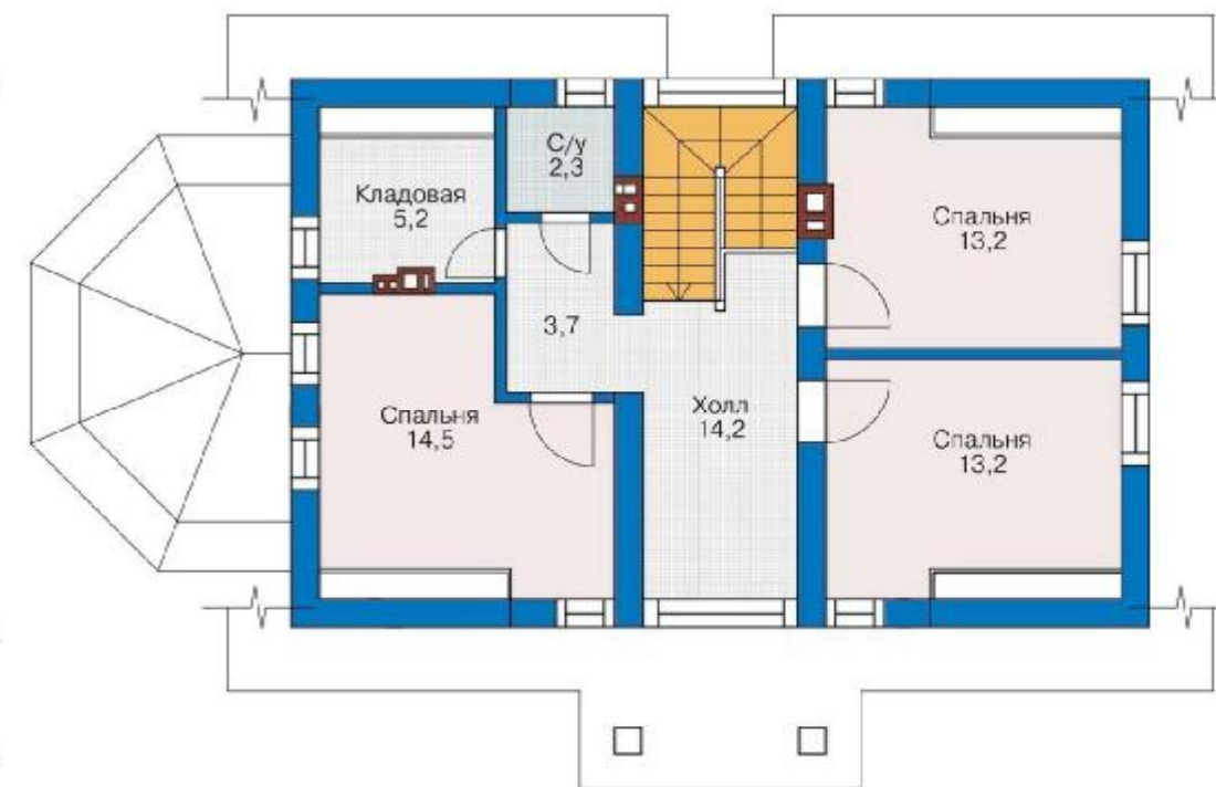
План мансардного этажа
