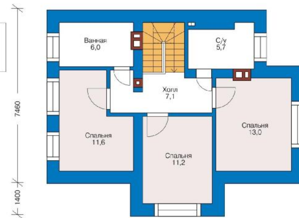
План мансардного этажа
