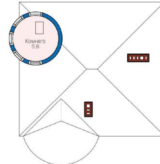
План мансардного этажа
