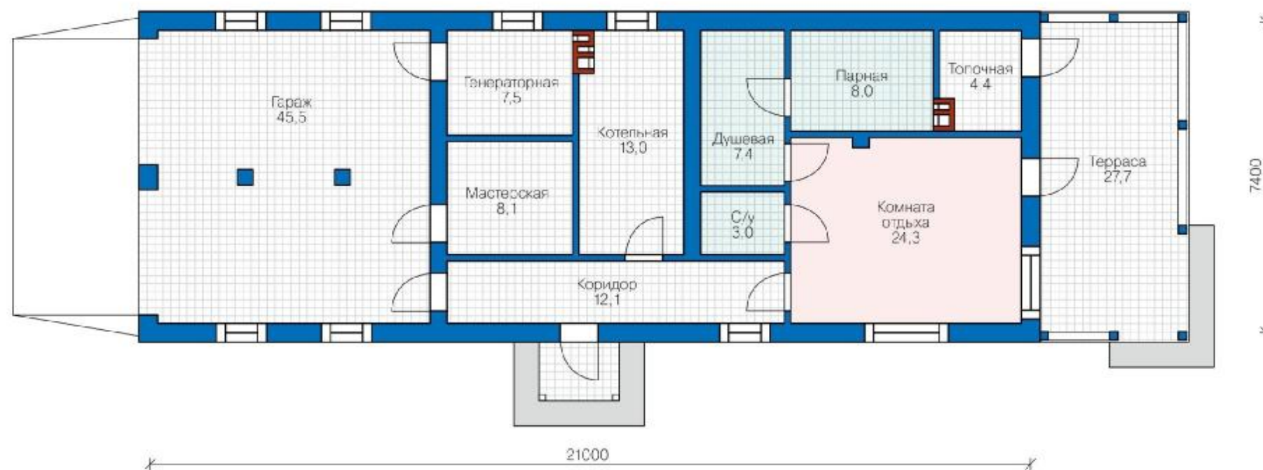
План первого этажа
